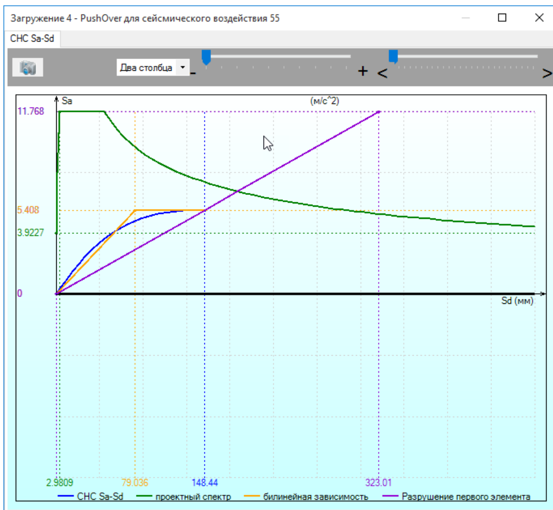
Рисунок 12.7 Результаты по Pushover для 55-го модуля
