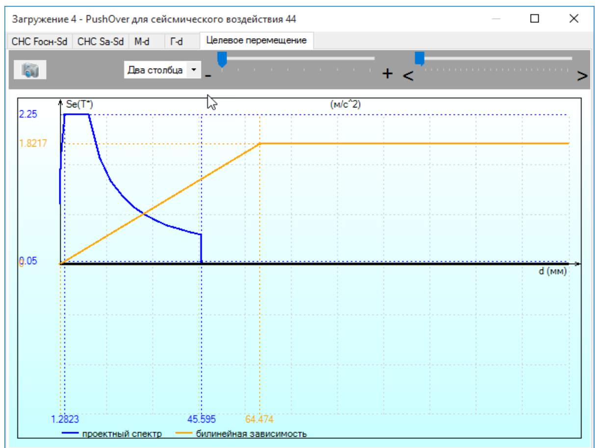
Рисунок 12.6 Результаты по Pushover для 44-го модуля
