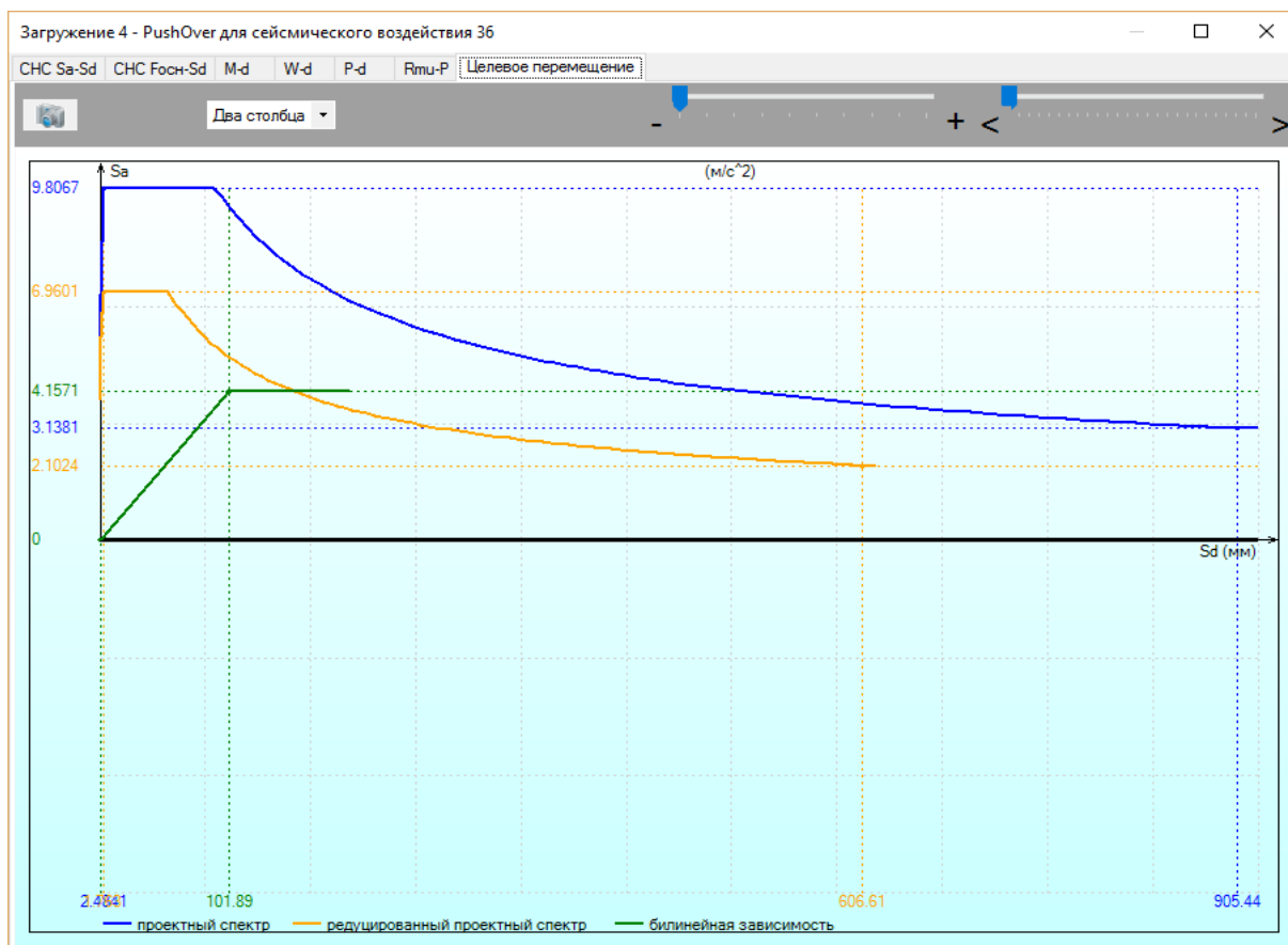
Рисунок 12.5 Результаты по Pushover для 36-го модуля
