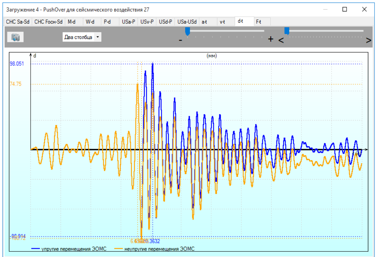
Рисунок 12.4 Результаты по Pushover для 27-го модуля
